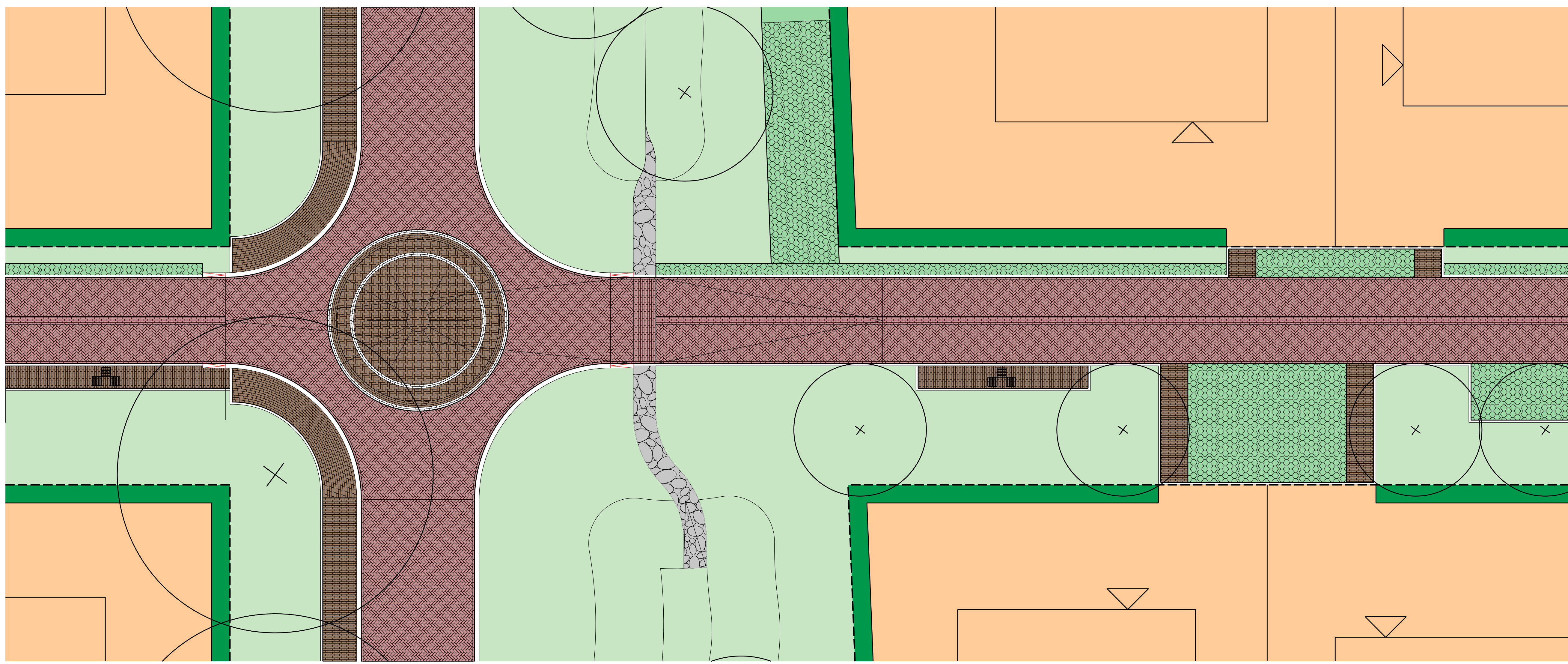
DETAILS schaal 1:100
