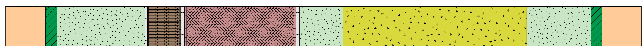
PROFIEL 1 schaal 1:100
