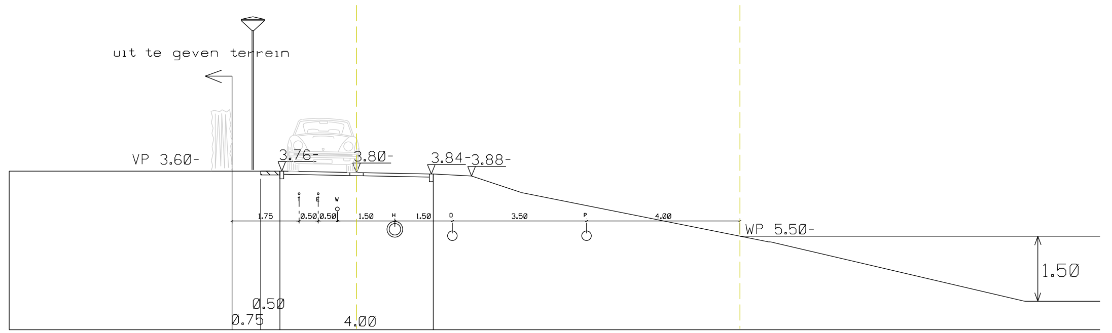
PROFIEL 4a schaal 1:100 (zonder parkeren)
