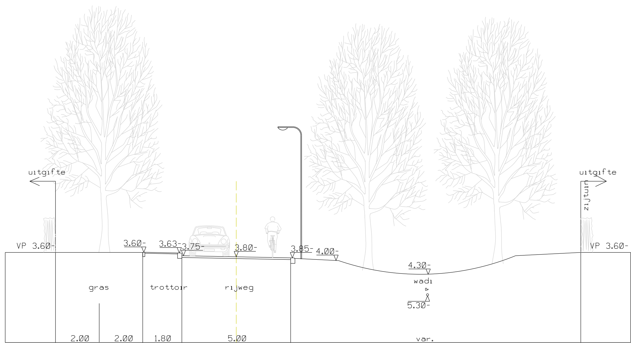
PROFIEL 1 schaal 1:100
