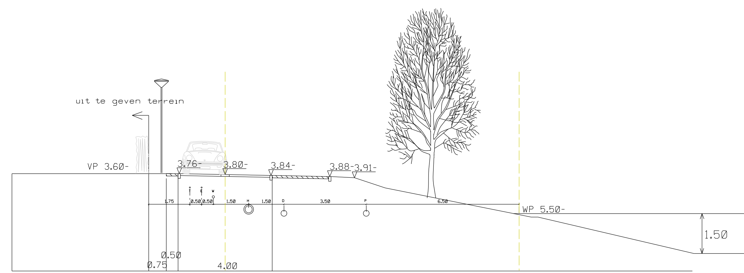
PROFIEL 4b schaal 1:100 (met parkeren)
