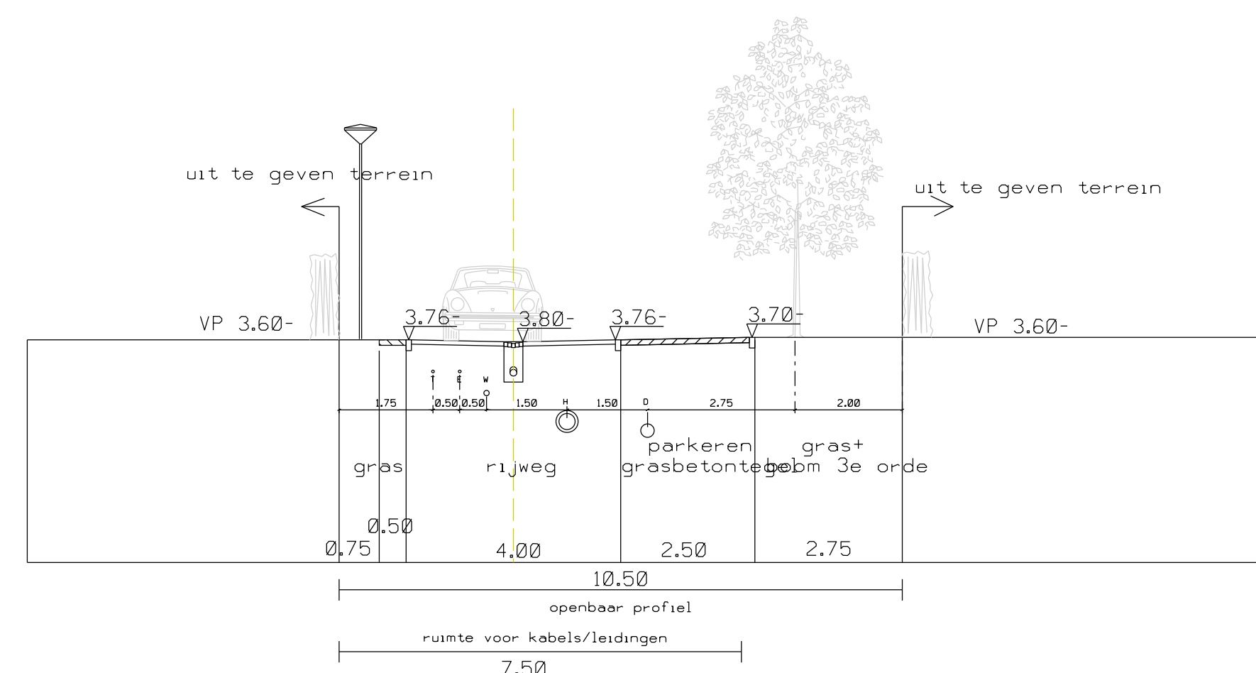
PROFIEL 2 schaal 1:100
