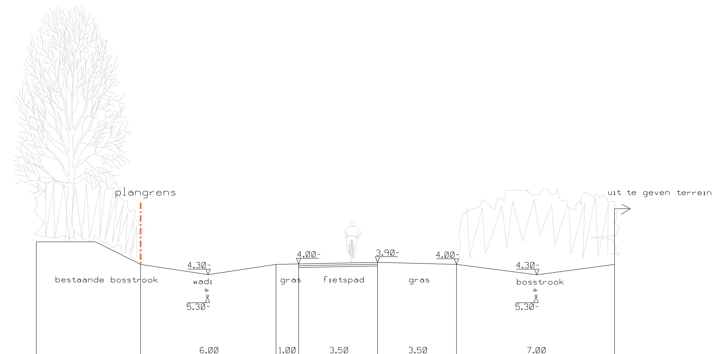
PROFIEL 3 schaal 1:100
